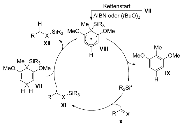
Schema 2. Radikalkettenreaktion der radikalischen Transferhydrosilylierung. \text{X} = \text{CH}_2 (Alkene) und \text{O} (Aldehyde). AIBN = Azobisisobutyronitril.
